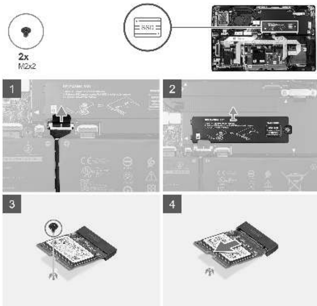
Abbildung 1. 2230-SSD
