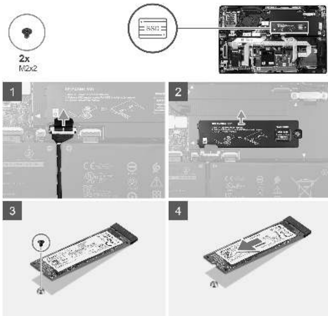
Abbildung 2. 2280-SSD
