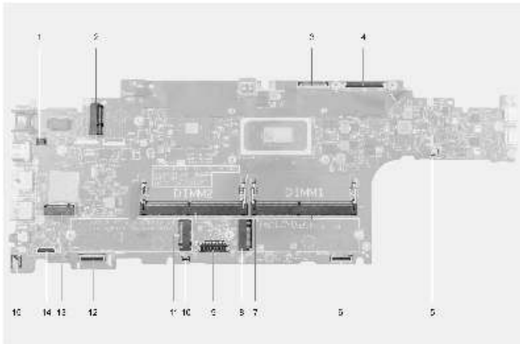
Abbildung 1. Systemplatinenanschlüsse
