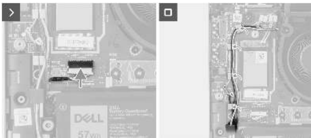
Abbildung 29. Installieren der Lautsprecher (Ultralight)
