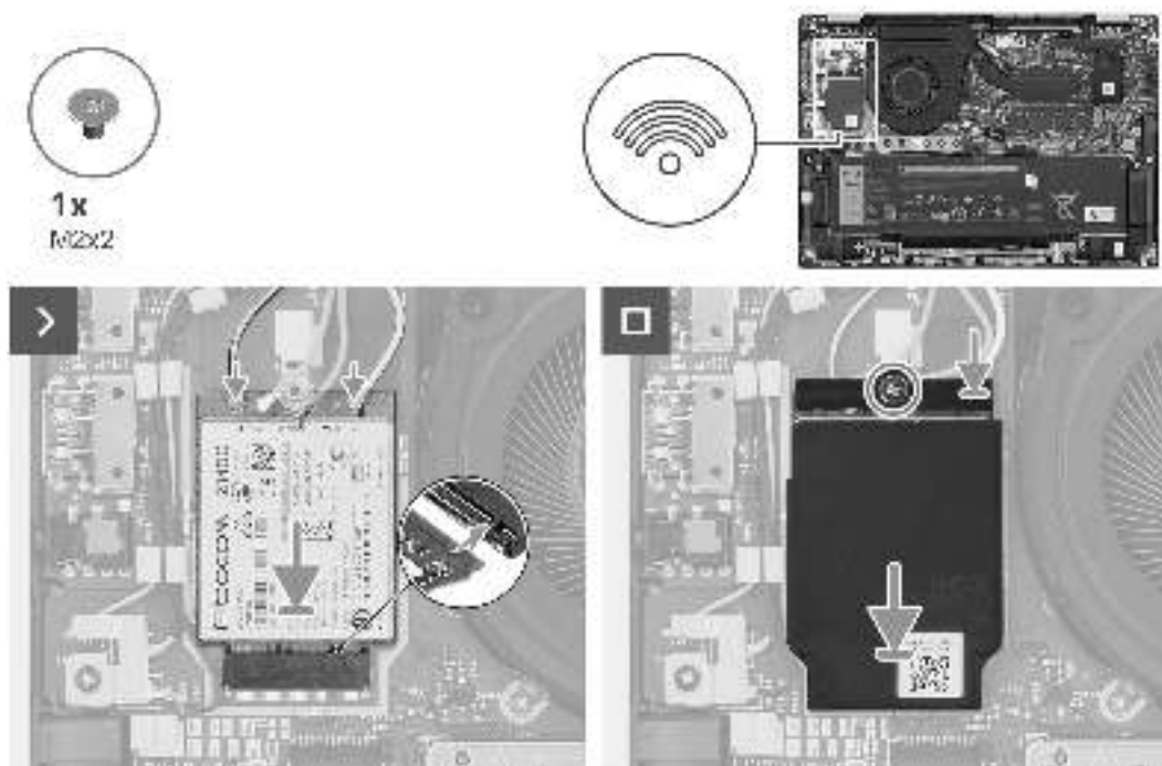
Abbildung 22. Installieren der 4G-WWAN-Karte
