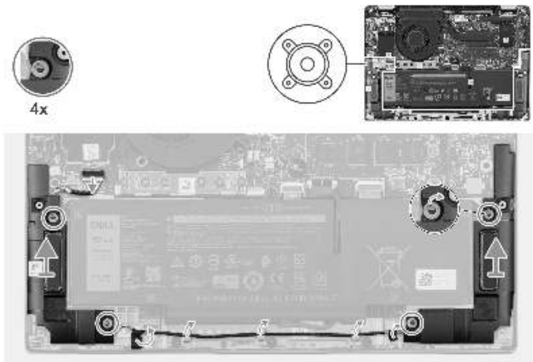
Abbildung 30. Entfernen der Lautsprecher für den Mainstream
