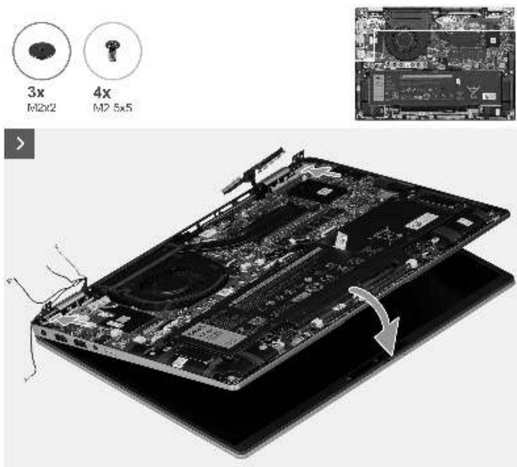
Abbildung 50. Installieren der Displaybaugruppe
