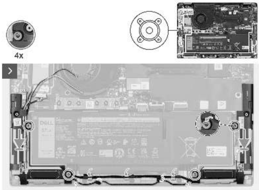
Abbildung 28. Installieren der Lautsprecher (Ultralight)
