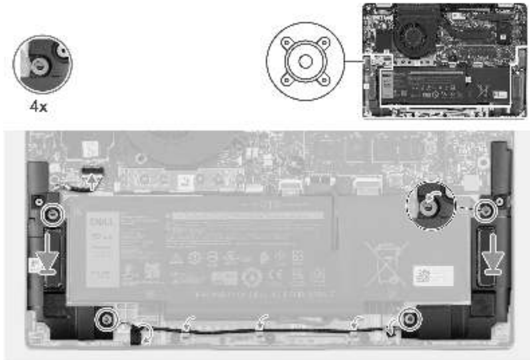
Abbildung 31. Installieren der Lautsprecher (Mainstream)
