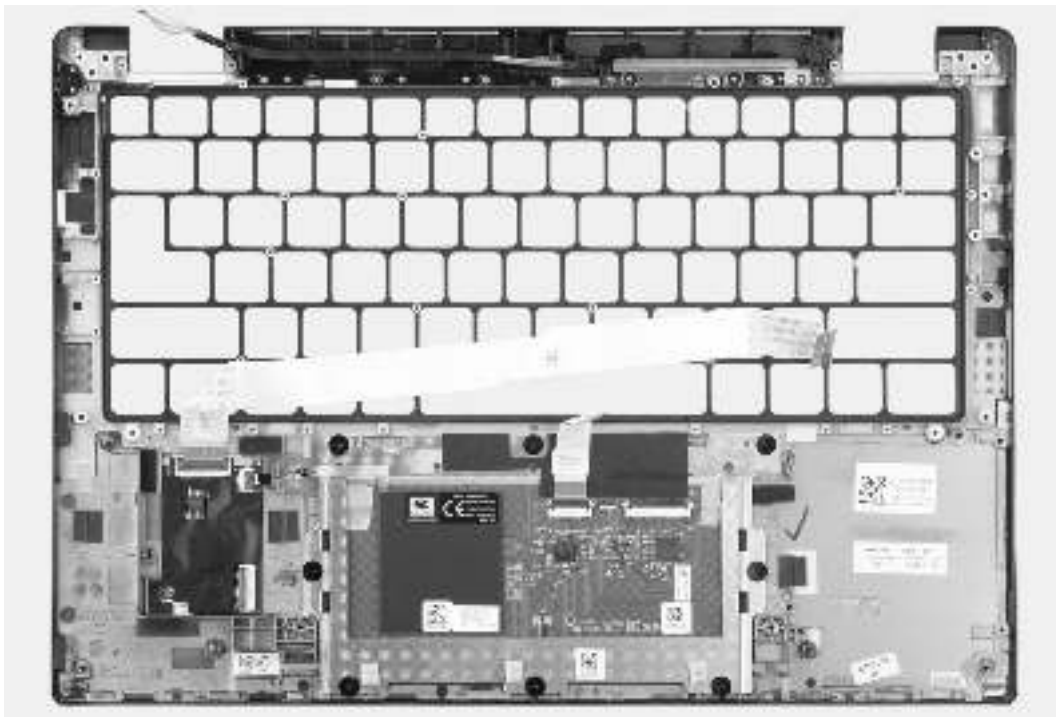
Abbildung 81. Entfernen der Handauflagenbaugruppe
