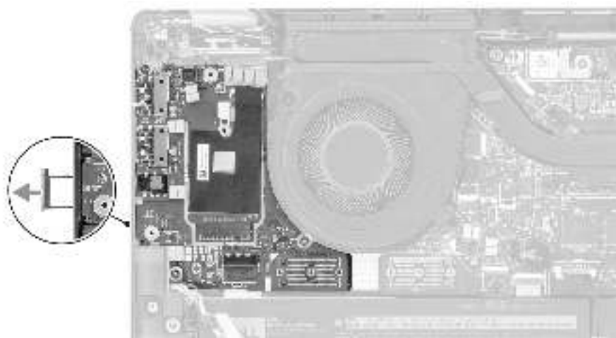
Abbildung 13. Entfernung der I/O-Zusatzplatine
