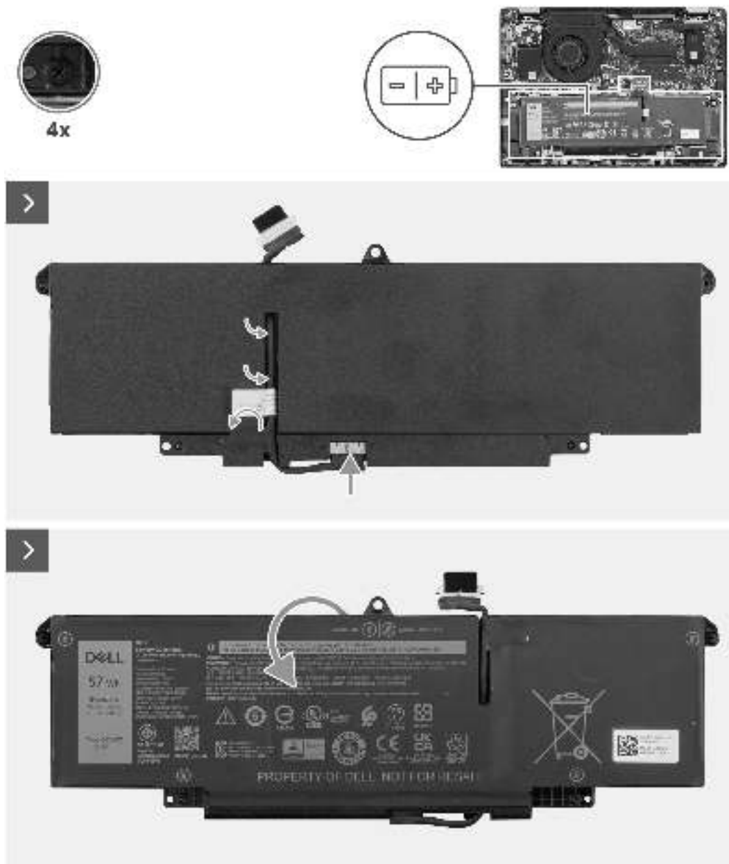
Abbildung 42. Installieren des Akkukabels
