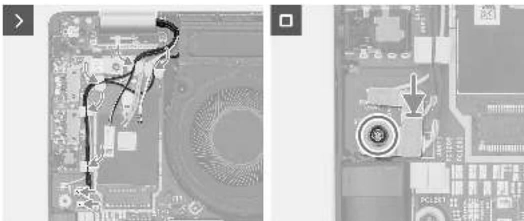
Abbildung 52. Installieren der Displaybaugruppe
