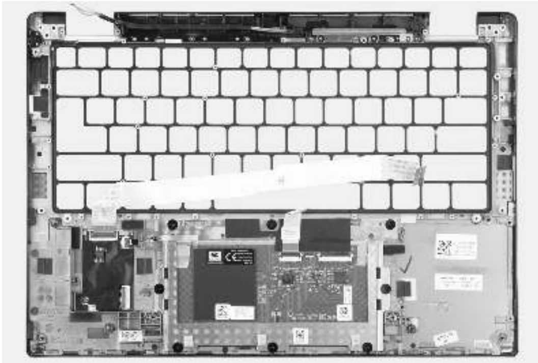
Abbildung 82. Installieren der Handauflagenbaugruppe
